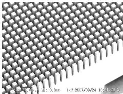
シリコン基板の溝入れ加工 (30 \mu\text{m} 幅)
